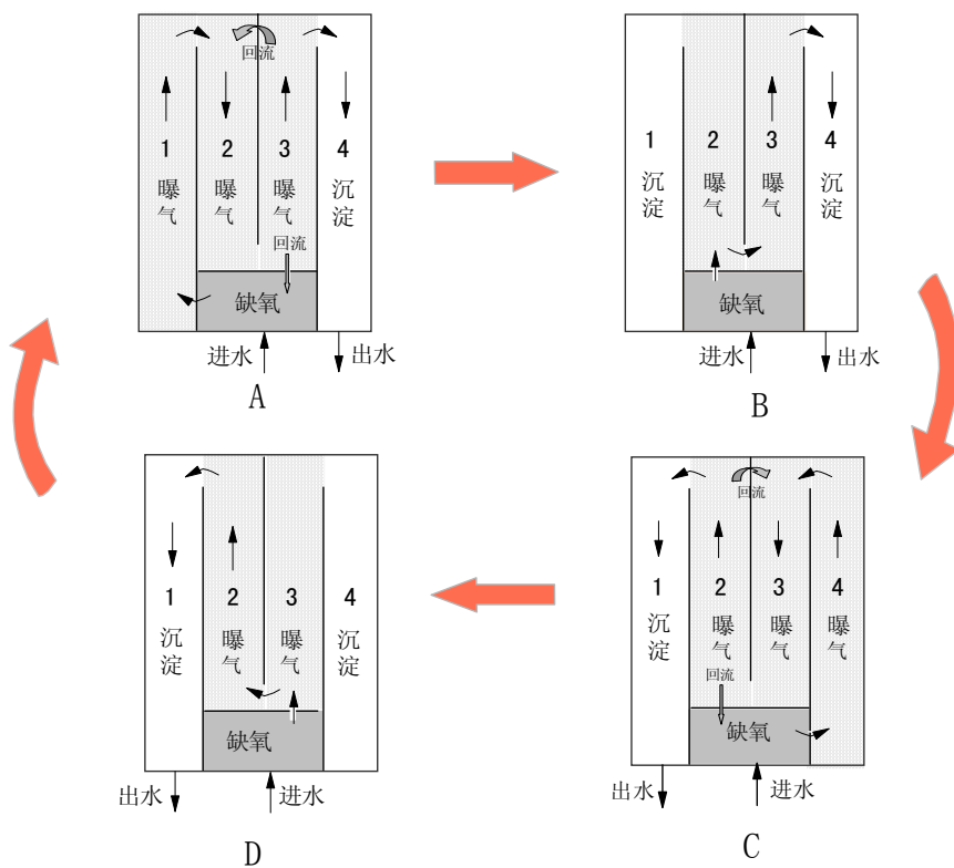
图 A.3 AICS 脱氮组合工艺流程
