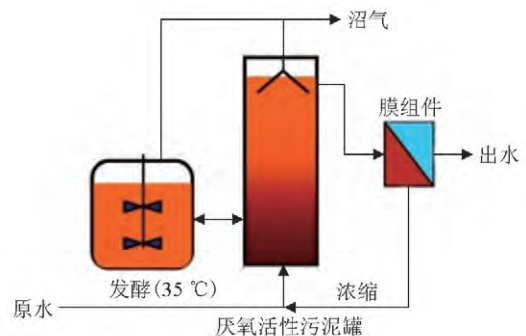
图 1 厌氧膜生物反应器结构示意图 Fig. 1 Schematic diagram of anaerobic membrane bioreactor
